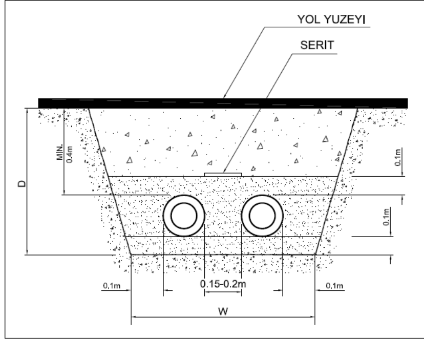
Şekil 2 - Kanal Kesiti
